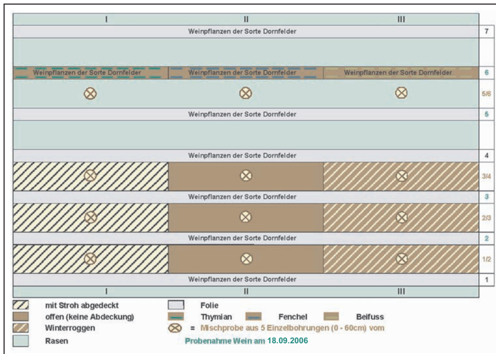
Abb. 1. Anordnung der Bepflanzung und Varianten bei einem Versuch auf dem Versuchsfeld des JKI in Berlin-Dahlem; Versuchsordnung 2006.
