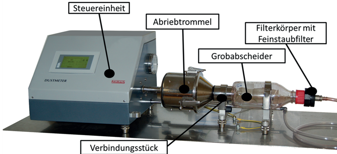
Abriebtrommel
